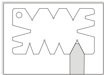
检测螺纹切削刀具的角度
